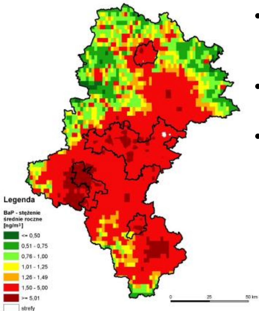
Rysunek 7.67. Rozkład przestrzenny wartości stężenia średniorocznego benzo(a)pirenu w pyłe PM10 w województwie śląskim w 2020 roku, opracowany z wykorzystaniem metody szacowania w oparciu o wyniki modelowania jakości powietrza dla roku 2020 wykonanego przez IOŚ-PIB [źródło: GIOŚ, IOŚ-PIB]
